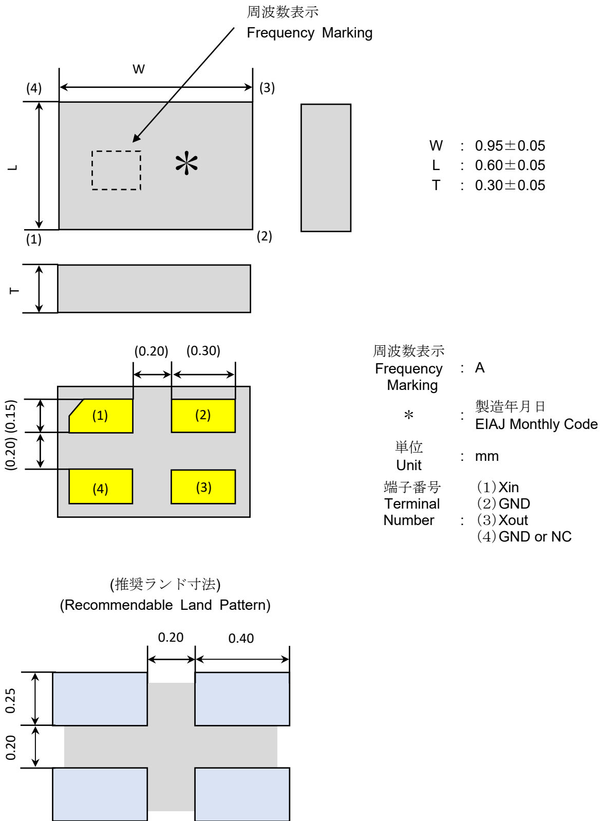
第1図 外形寸法図 Figure 1. Dimensions
